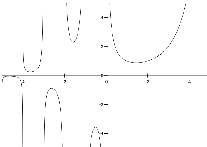
Abbildung 3.7: Die Gammafunktion \Gamma(x)
