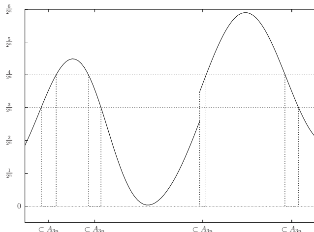
Abbildung 6.2: Lebesgue-Integration
